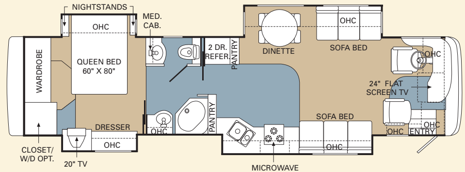
40' PDQ Floorplan
